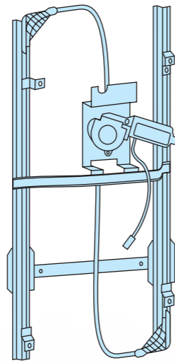
385/174 d-rh-rechts 385/175 s-lh-links elettrico con motorino electric with motor elektrisch mit Motor
